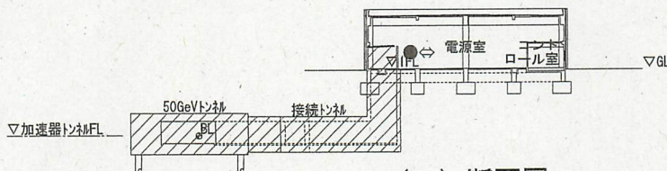
(b) 断面図
