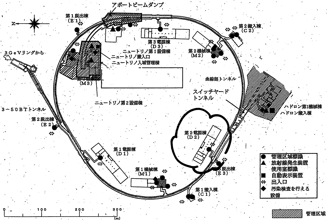
50GeVシンクロトロン施設
