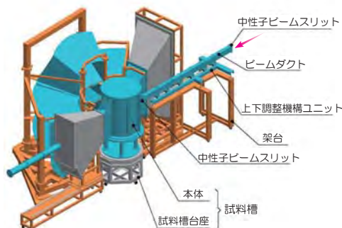
特殊環境中性子回折装置「SPICA」/BLO9 完成予想図(MLF 東側の増設建屋に設置)
