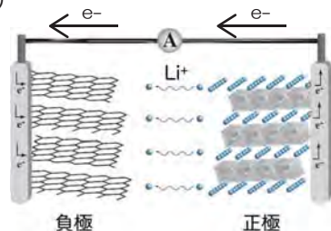
Liイオン蓄電池の構造
